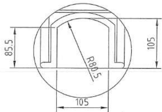
DETALLE A ESCALA 1:5
