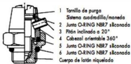
Purgador Manual "MPS" 1/8"
