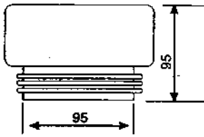
CONCENTRICO
