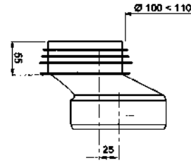
MAXI EXCENTRICO
