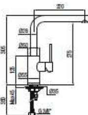
Monomando fregadero vertical MAX-TRES
