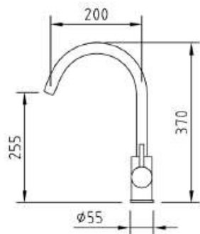
98522 Fregadero Inox Right
